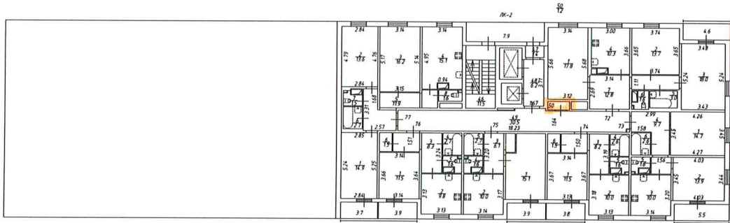
План 9 этажа н. 272
